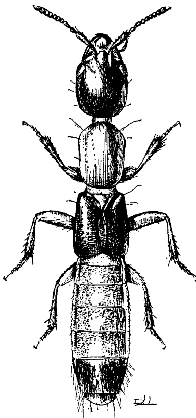
13. ábra. Xantholinus decorus ERICHSON ♂ (Eredeti)
