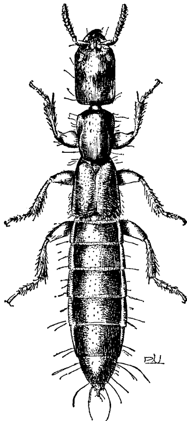
4. ábra. Metoponcus brevicornis (ERICHSON) ♂ (Eredeti)
