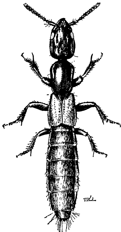
9. ábra. Gauropterus fulgidus (FABRICIUS) ♂ (Eredeti)
