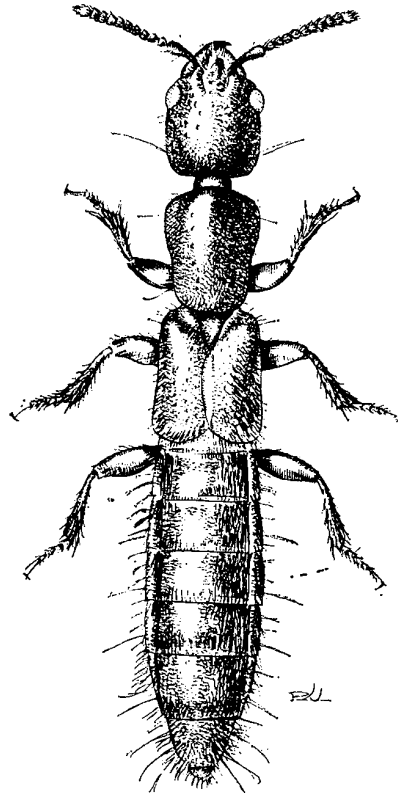
10. ábra. Nudobius lentus (GRAVENHORST) ♂ (Eredeti)
