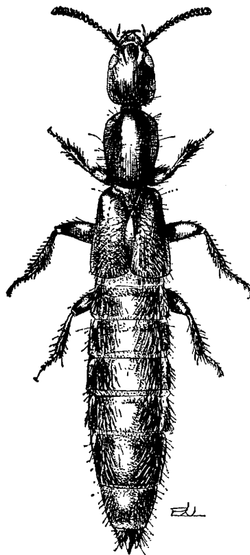
11. ábra. Gyrohypnus fracticornis (O. F. MÜLLER) ♂ (Eredeti)
