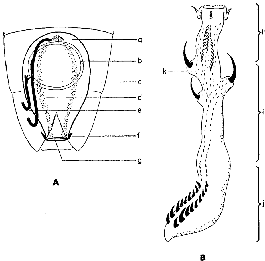
3. ábra. A: Xantholinus sp. ♂ ivarszerve — A: aedoeagus ( a = bulbus basalis, b = operculum, c = saccus internus, d = ductus ejaculatorius, e = trachea, f = parameron és g = ivarnyílás) és B: a belső zsák külön, kifordítva ( h = portio distalis, i = portio intermedia, j = portio proxima, k = pars caeca) (A: BORODNI, B: COIFFAIT nyomán, kissé módosítva)
