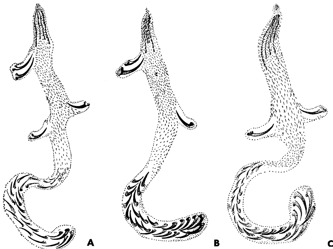
16. ábra. A: Xantholinus lichtneckerti TÓTH, B: X. magyareicus TÓTH és C: X. pseudobalaton TÓTH ♂ ivarszervének belső zsákja (A—C: TÓTH nyomán)
