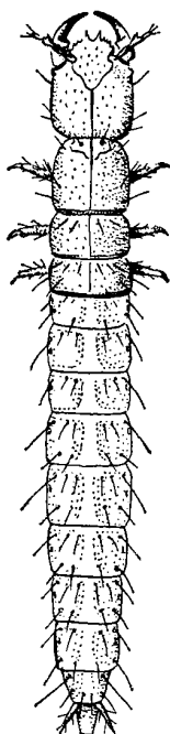
1. ábra. Xantholinus tricolor (FABRICIUS) lárva (POTOCKAJA nyomán)
