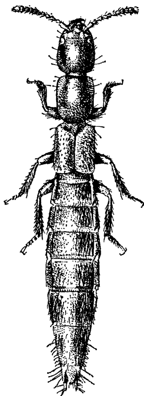
19. ábra. Othius punctulatus (GOEZE) ♂ (Eredeti)
