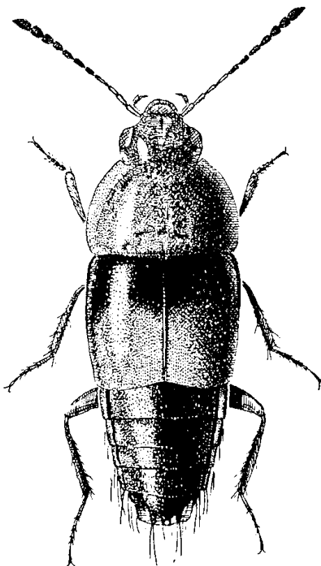
13. ábra. Tachyporus obtusus (LINNAEUS) ♂ (SZÉKESSY nyomán)
