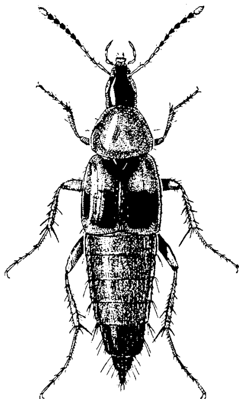
11. ábra. Bolitobius lunulatus (LINNAEUS) ♀ (SZÉKESSY nyomán)
