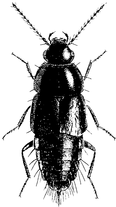
2. ábra. Habrocerus capillaricornis (GRAVENHORST) ♀ (SZÉKESY nyomán)
