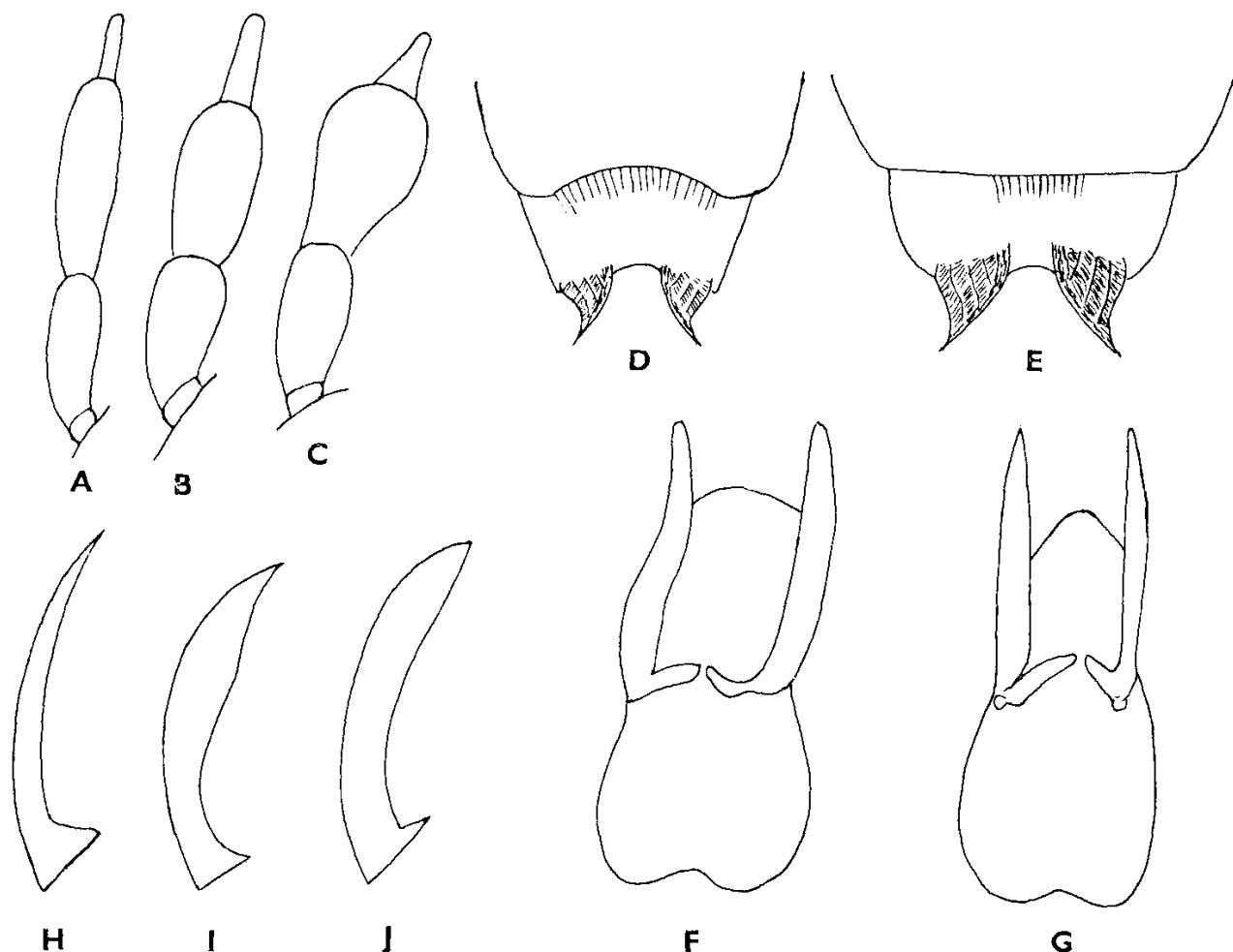
7. ábra. A—C: Mycetoporus fajcsoportok állkapcsi tapogatói — D: M. splendidus (GRAVENHORST) és E: M. longicornis MAEKLIN potrohcsúcsa alulnézetben — F: M. monticola FOWLER és G: M. baudueri MULSANT & REY ♂ ivarszerve alulnézetben — H: M. longulus MANNERHEIM, I: M. ruficornis KRAATZ és J: M. brunneus (MARSHAM) ♂ ivarszervének parameronja felülnézetben (A—E: HANSEN, F—J: LOHSE nyomán)
