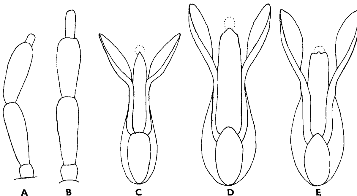
14. ábra. A: Tachyporus nitidulus (FABRICIUS) és B: T. solutus ERICHSON állkapcsi tapogatója — C: T. atriceps STEPHENS, D: T. ruficollis GRAVENHORST és E: T. signifer PANDELLÉ ♂ ivarszerve alulnézetben (A—E: LOHSE nyomán)
