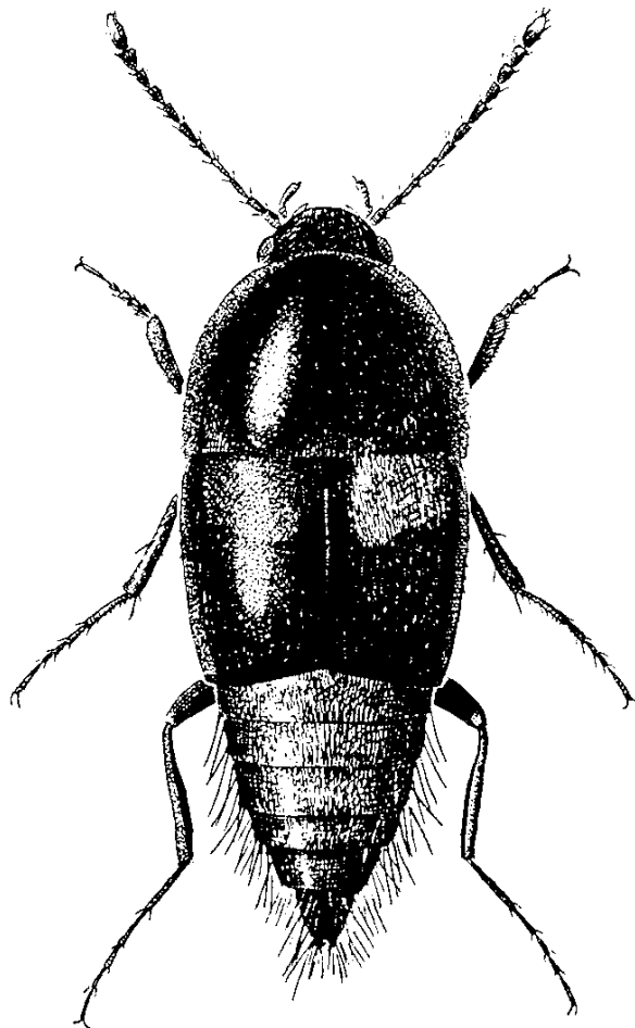
24. ábra. Sepedophilus bipustulatus (GRAVENHORST) ♂ (SZÉKESSY nyomán)
