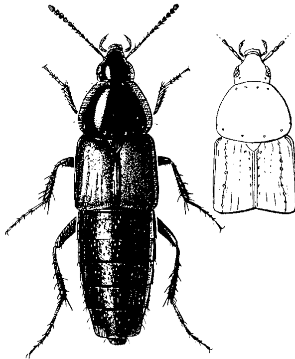
5. ábra. Mycetoporus splendens (MARSHAM) ♀ (SZÉKESSY nyomán)
