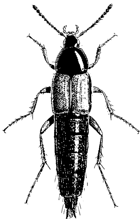
8. ábra. Bryocharis analis (PAYKULL) ♀ (SZÉKESY nyomán)
