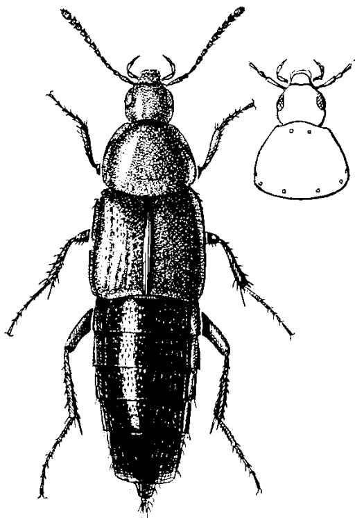
10. ábra. Bryoporus rufus (ERICHSON) ♀ (SZÉKESY nyomán)
