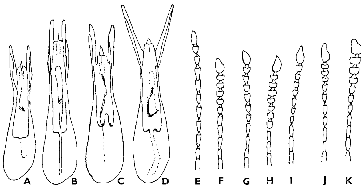
26. ábra. A: Sepedophilus testaceus (FABRICIUS), B: S. marshami (STEPHENS), C: S. strigosus (J. SAHLBERG) és D: S. lokayi SMETANA ♂ ivarszerve alulnézetben — E: S. littoreus (LINNAEUS), F: S. testaceus (FABRICIUS), G: S. marshami (STEPHENS), H: S. bipunctatus (GRAVENHORST), I: S. pedicularius (GRAVENHORST), J: S. nigripennis (STEPHENS) és K: S. immaculatus (STEPHENS) csápja (A—D: SMETANA, E—K: HAMMOND nyomán)
