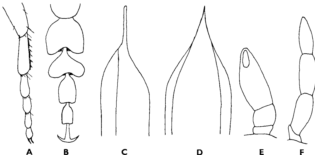
9. ábra. A: Bryocharis analis (PAYKULL) elülső lábfeje oldalnézetben — B: B. inclinans (GRAVENHORST) ♂ elülső lábfeje felülnézetben, C: ♂ ivarszervének csúcsa oldal- és D: alulnézetben — E: Bryocharis sp. ajaktapogatója és F: állkapcsi tapogatója oldalnézetben (A és E—F: HANSEN, B—D: FAGEL nyomán)
