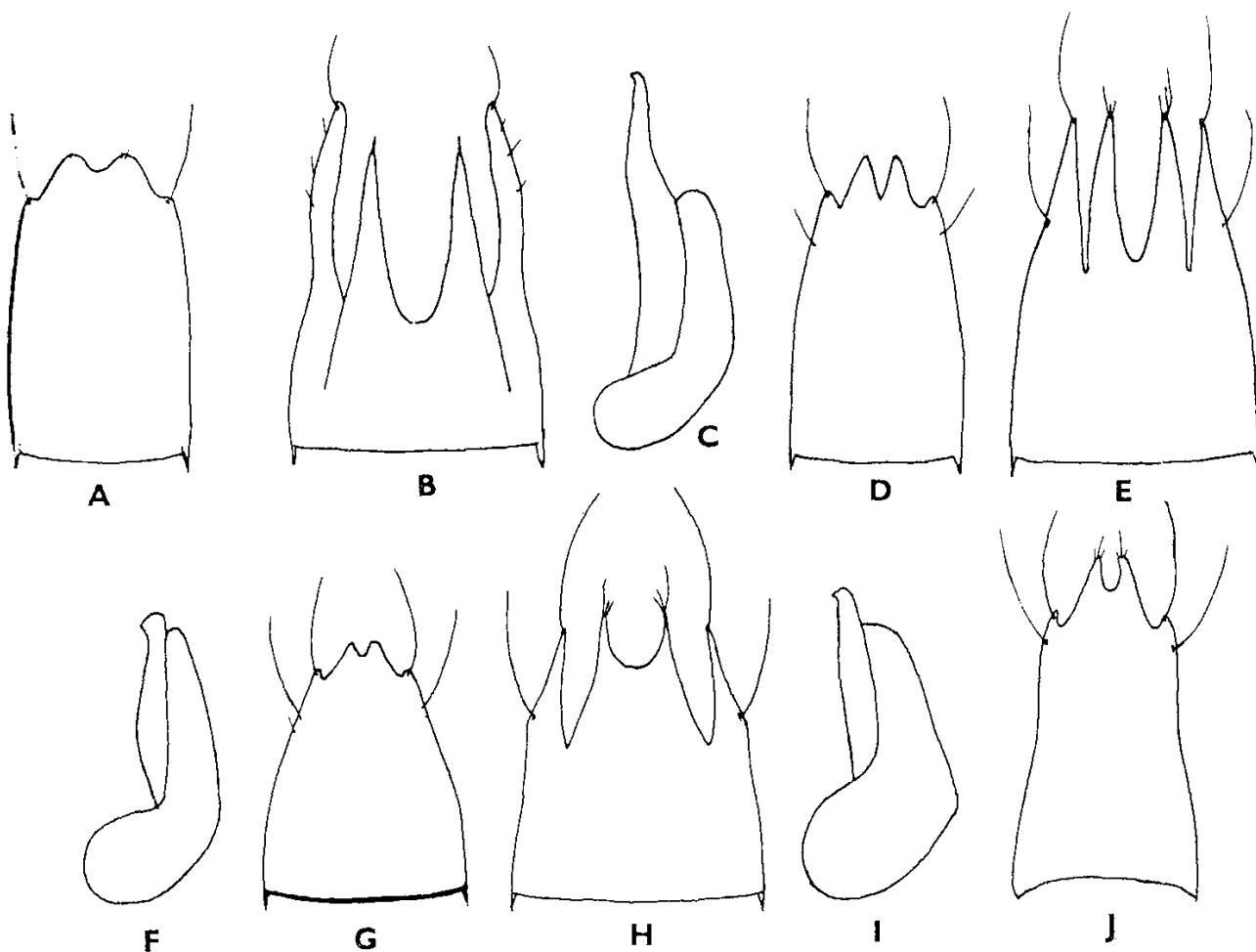
19. ábra. A—C: Tachinus subterraneus (LINNAEUS), D—F: T. fimetarius GRAVENHORST, G—I: T. bonvouloiri PANDELLE, J: T. scapularis STEPHENS, [A, D, G, J: a ♂ és B, E, H: a ♀ potrohának 8. (6. látható) hátlemeze felülnézetben, valamint C, F, I: a ♂ ivarszerve oldalnézetben] (A—J: ULLRICH nyomán)
