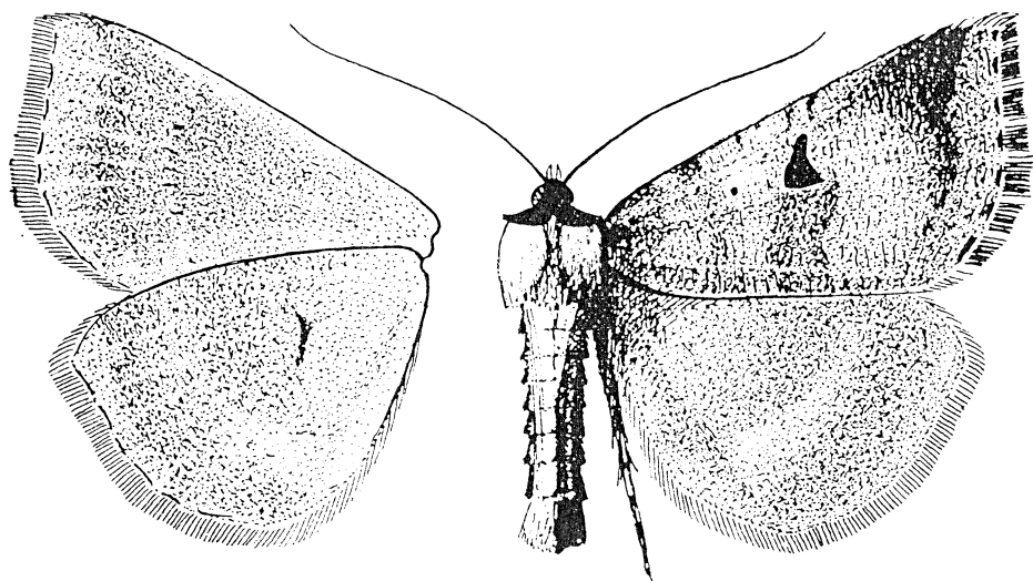
34. ábra. Lygephila lusoria L. ssp. fusca KYSELA ♂ (Eredeti)
