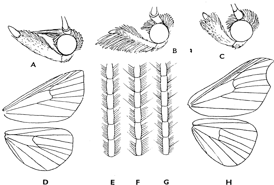
22. ábra. A: Colobochyla , B: Rivula és C: Laspeyria feje — D: Colobochyla szárnyerezete — E: Colobochyla , F: Rivula és G: Laspeyria hím csáppostorának részlete — H: Laspeyria szárnyerezete (Eredeti)
