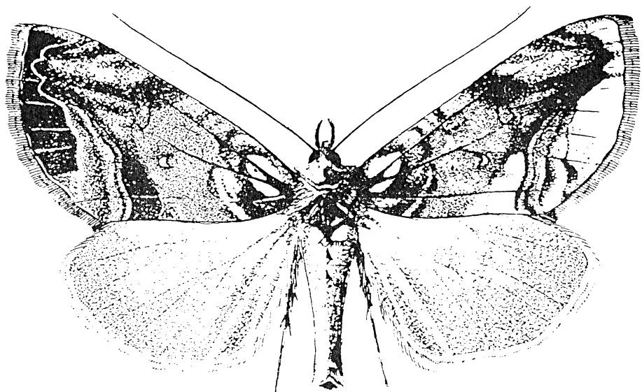
65. ábra. Chrysoptera c-aureum KNÖCH ♂ (Eredeti)
