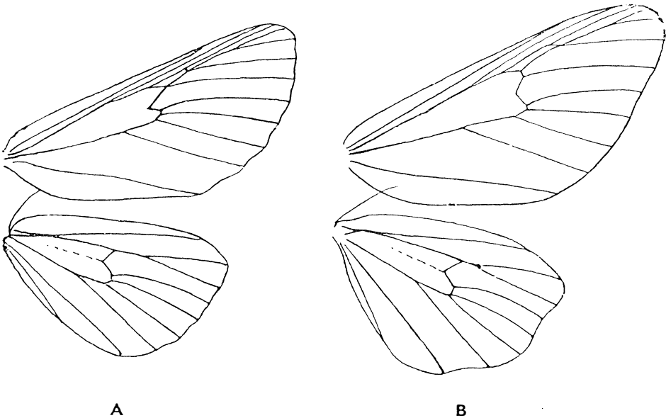
78. ábra. A: Episema és B: Panthea szárnyerezete (Eredeti)
