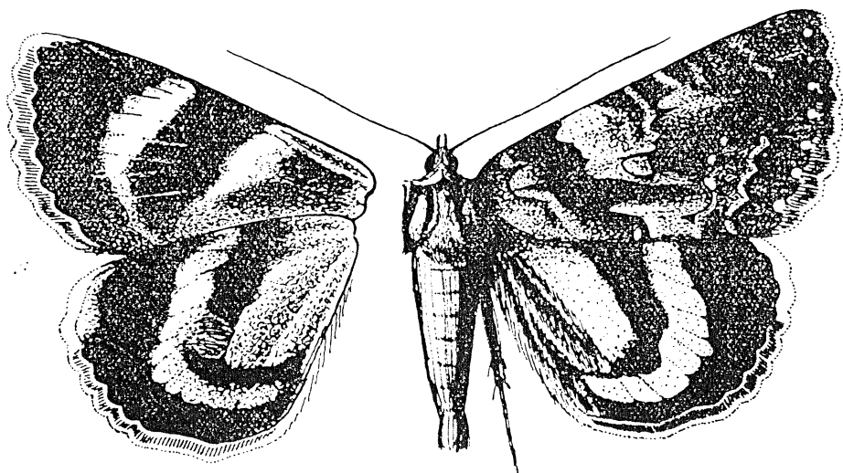
42. ábra. Ephesia diversa Hbn. ♂ (Eredeti)
