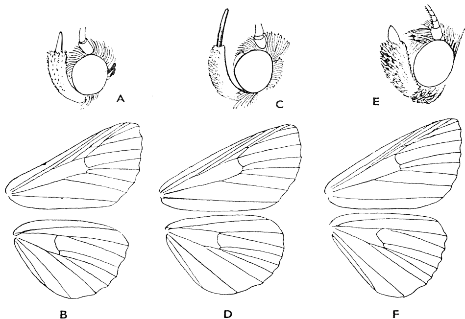
39. ábra. A—B: Aedia . C—D: Catephia és E—F: Catocala feje és szárnyerezete (Eredeti)
