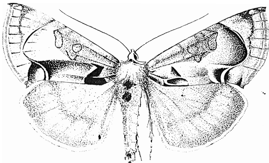
60. ábra. Plusia zosimi HBN. ♂ (Eredeti)
