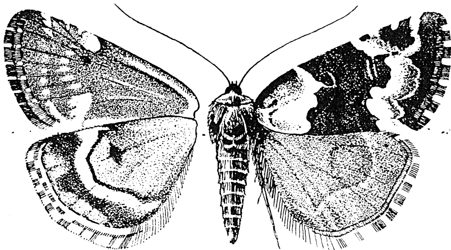
100. ábra. Jaspidia deceptor Sc. ♂ (Eredeti)
