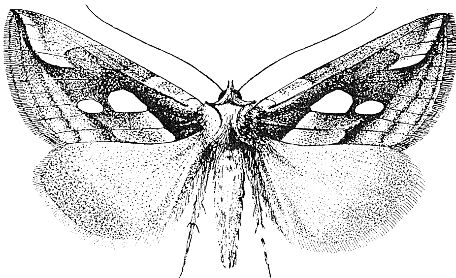
67. ábra. Chrysaspidia festucae L. ♂ (Eredeti)
