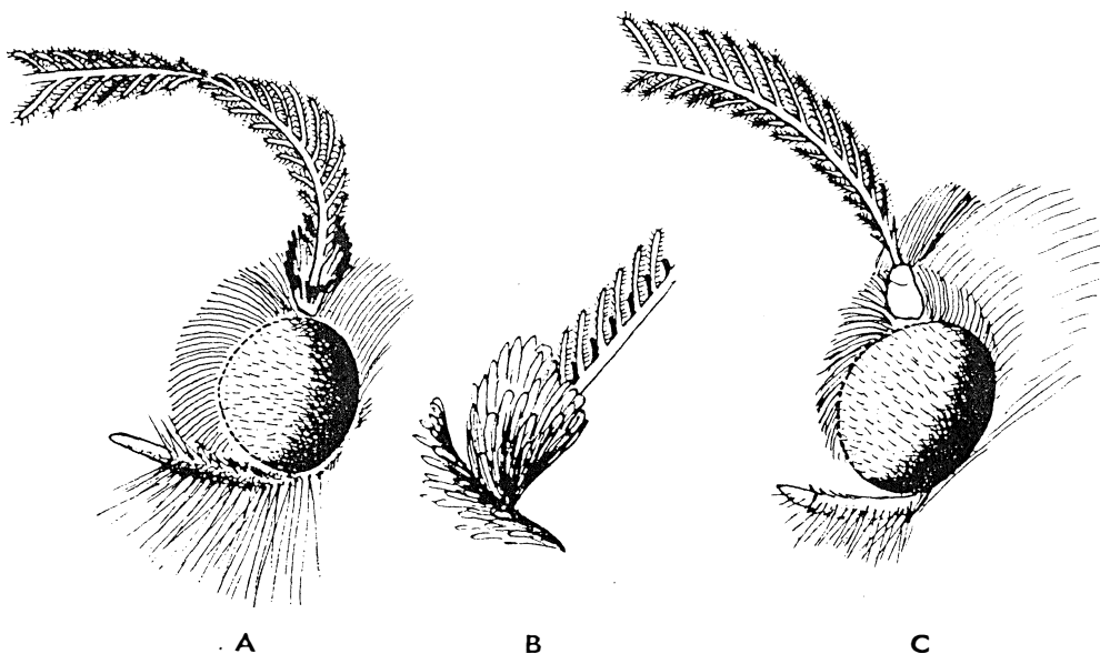
77. ábra. A: Episema feje oldalról és B: csáptöve felülről — C: Panthea feje (Eredeti)
