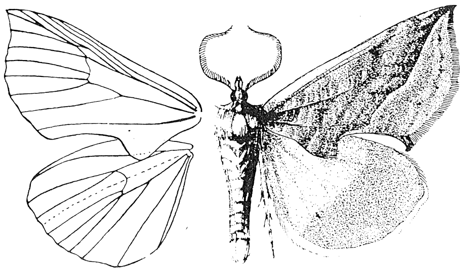
56. ábra. Calpe thalictri BKH. ♂ és szárnyerezete (Eredeti)
