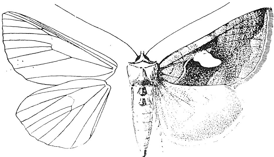
68. ábra. Chrysaspidia bractea SCHIFF. ♂ és szárnyerezete (Eredeti)
