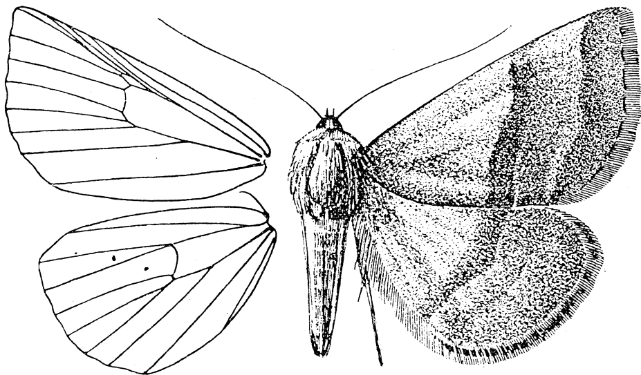
102. ábra. Prothymia viridaria CL. ♂ és szárnyerezete (Eredeti)
