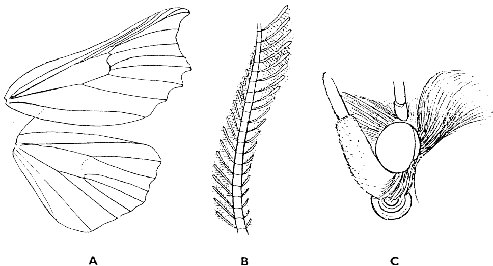
54. ábra. Scoliopteryx libatrix L. A: erezete. B: hím csápostorának részlete és C: feje (Eredeti)
