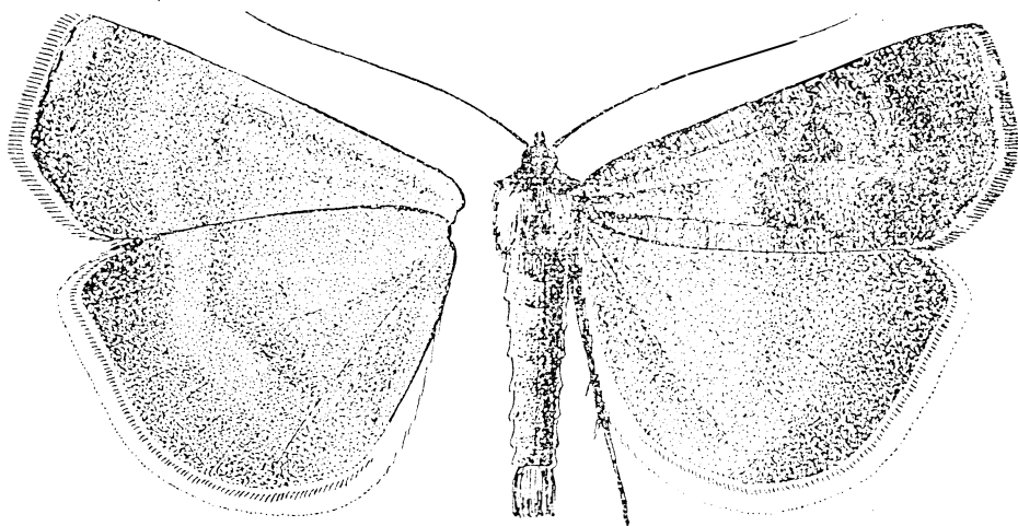
33. ábra. Eccrita ludicra HBN. ♂ (Eredeti)
