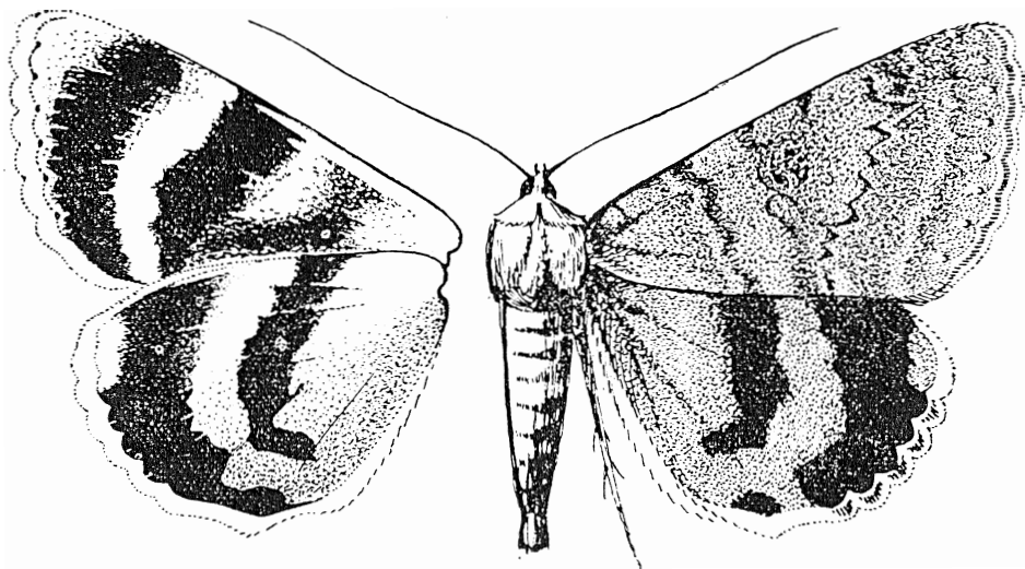
47. ábra. Catocala puerpera GIORNA ♂ (Eredeti)
