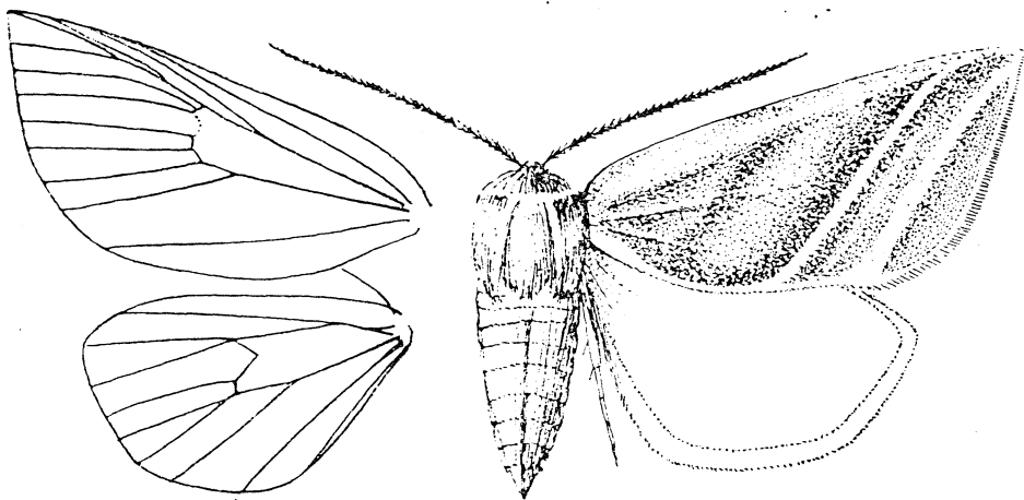
83. ábra. Hylophila fagana F. ♀ és szárnyerezete (Eredeti)
