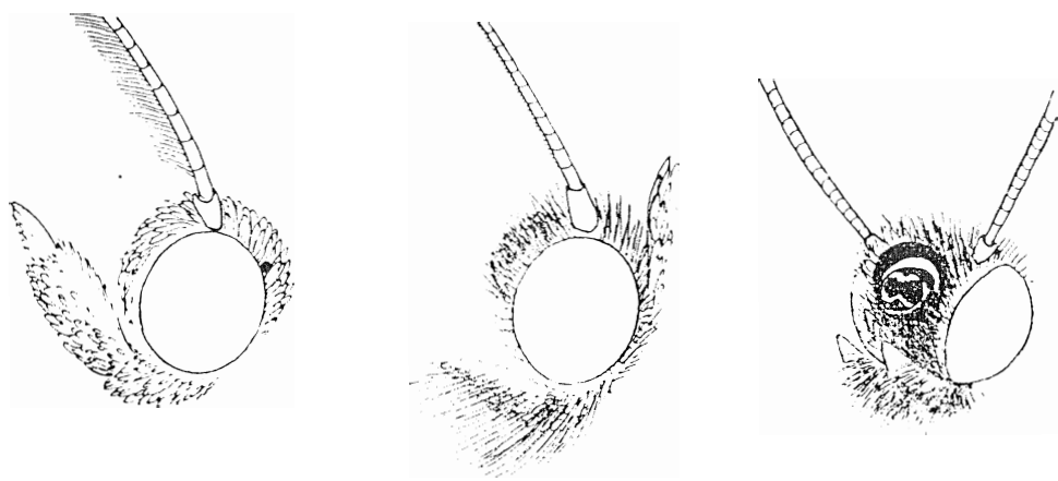
111. ábra. A: Leptosia . B: Panemeria és C: Apaustis feje (Eredeti)
