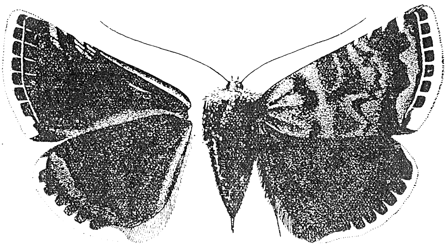
113. ábra. Apantesis rupicola SCHIFF. 2 (Eredeti)
