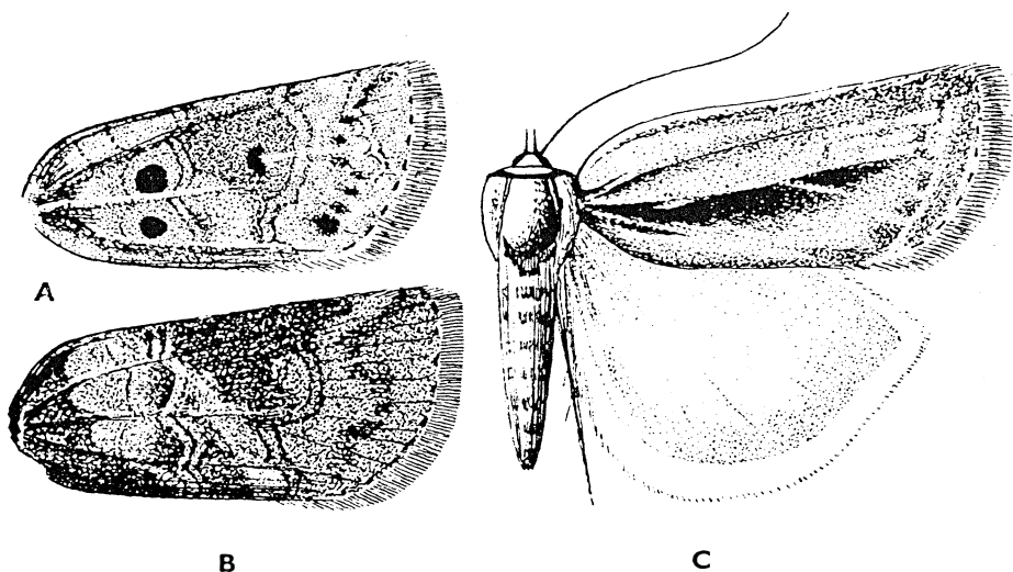
89. ábra. A–C: Nycteola Revayana Sc. ♂ különféle formái (Eredeti)
