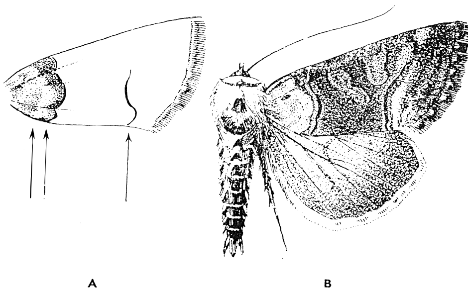
72. ábra. A: Abrostola trigemina WERNB. elülső szárnyának tőttere és külső keresztvonalának alsó fele (részletrajz) — B: A. asclepiadis SCHIFF. ♂ (Eredeti)
