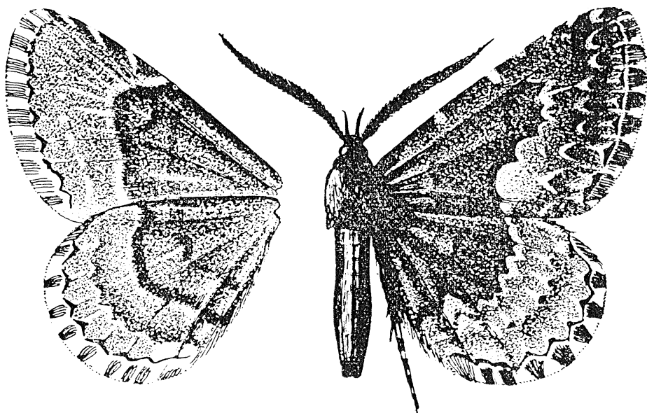
20. ábra. Parascotia fuliginaria L. ♂ (Eredeti)
