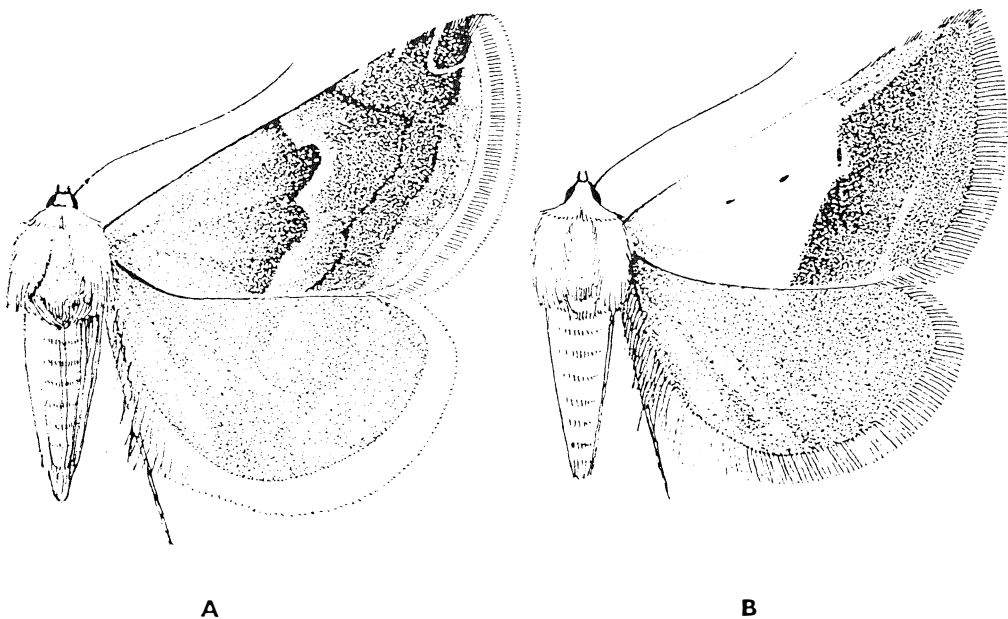
104. ábra. A: Porphyrinia rosea HBN. ♀ és B: P. pannonica Frr. ♂ (Eredeti)
