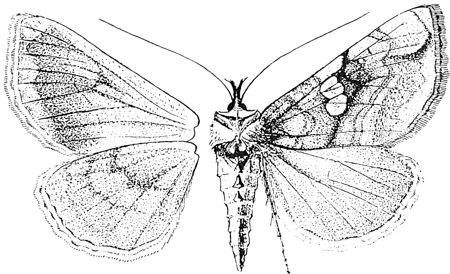
63. ábra. Polychrysis moneta F. ♀ (Eredeti)
