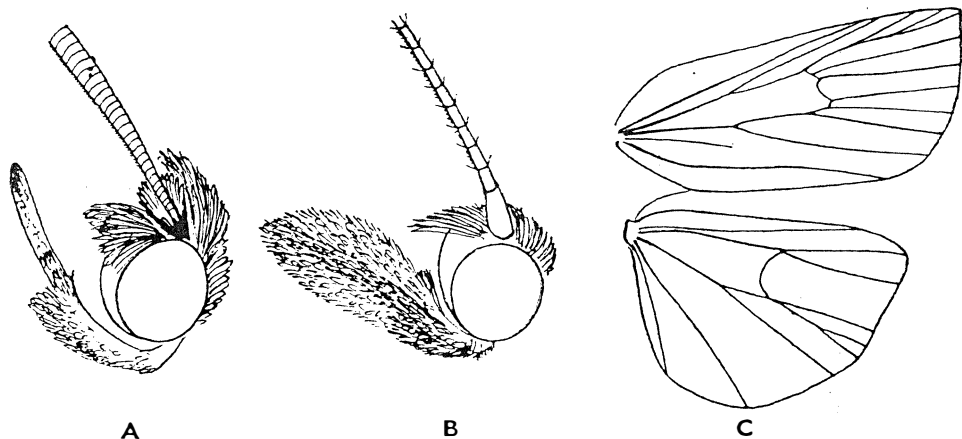
87. ábra. A: Eutelia és B: Nycteola feje — C: Nycteola szárnyereztete (Eredeti)
