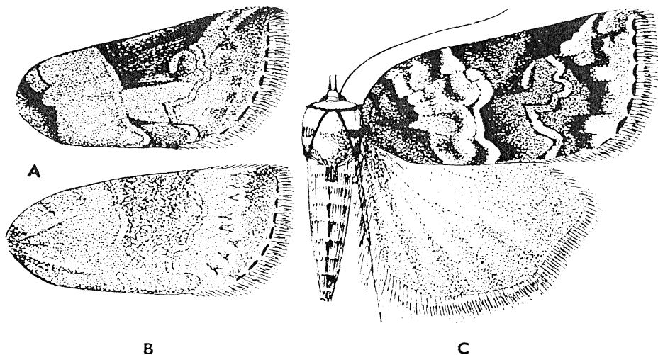
88. ábra. A: Nycteola siculana FUCHS és B: N. asiatica KRUL. elülső szárnya — C: N. degenerana HBN. ♂ (Eredeti)
