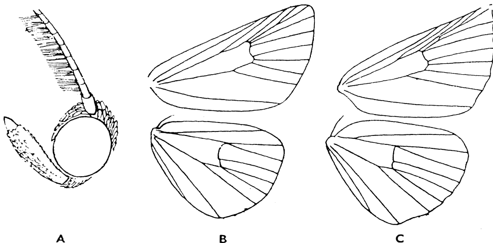
108. ábra. A: Eublemma feje — B: Panemeria és C: Apaustis szárnyerezete (Eredeti)
