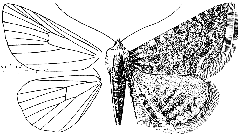
110. ábra. Leptosia Dardouini B. ♂ és szárnyerezete (Eredeti)
