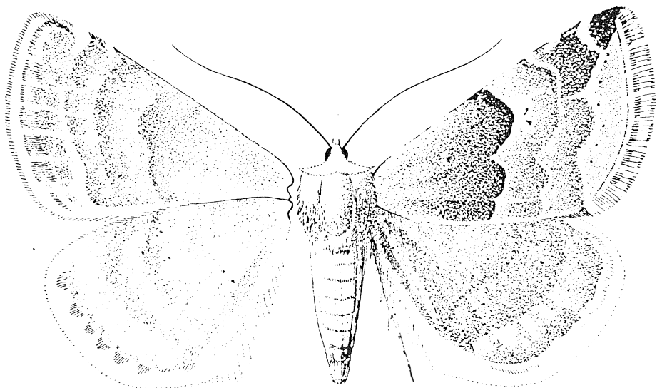
105. ábra. Porphyria respersa HBN. 2 (Eredeti)
