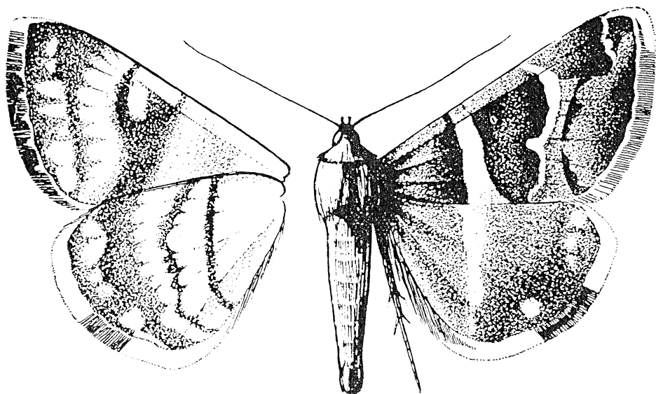
31. ábra. Grammodes stolidus F. ♂ (Eredeti)
