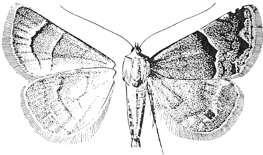
109. ábra. Eublemma arcuina HBN. ♂ (Eredeti)
