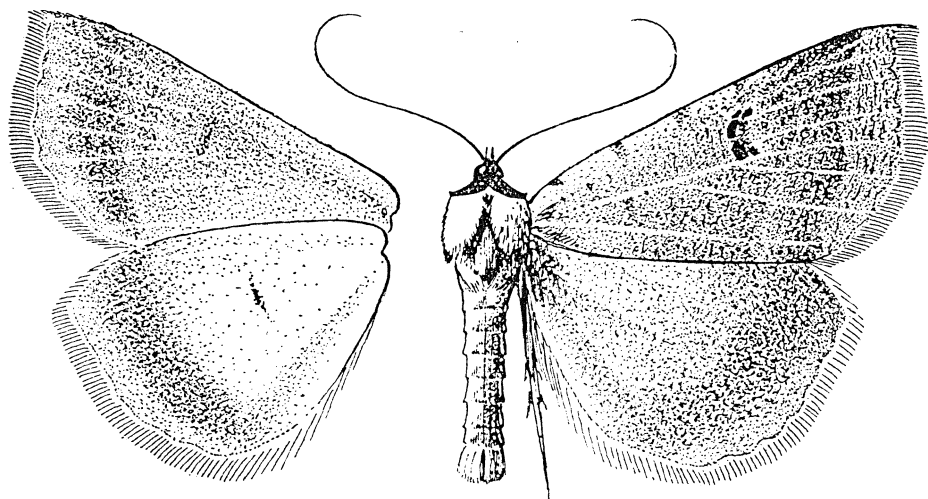
35. ábra. Lygephila cracca F. ♂ (Eredeti)
