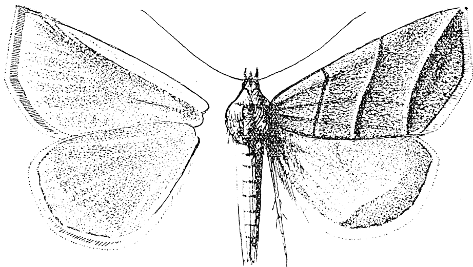
24. ábra. Colobochyla salicalis SCHIFF ♂ (Eredeti)
