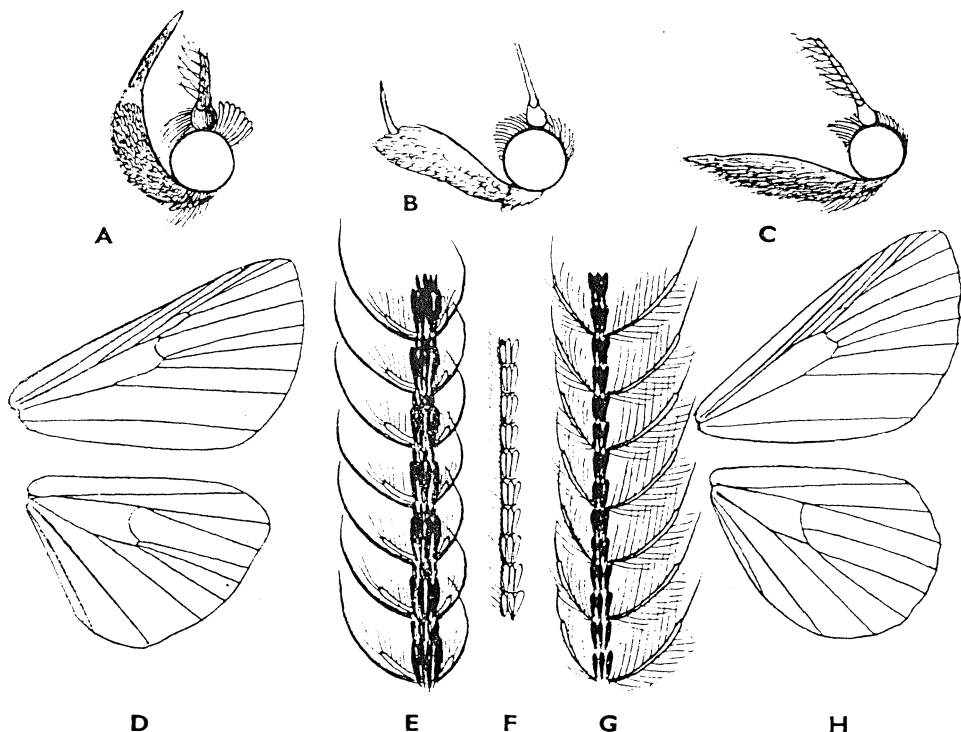
18. ábra. A: Epizeuxis , B: Orectis és C: Parascotia feje — D: Epizeuxis szárnyerezete és E: hím csápotorának részlete — F: Orectis proboscidata HS. és G: Parascotia fuliginaria L. hím csápotorának részlete — H: Parascotia szárnyerezete (Eredeti)
