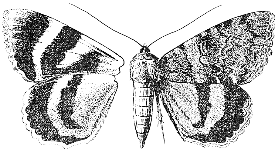
48. ábra. Catocala elocata Esp. ♀ (Eredeti)
