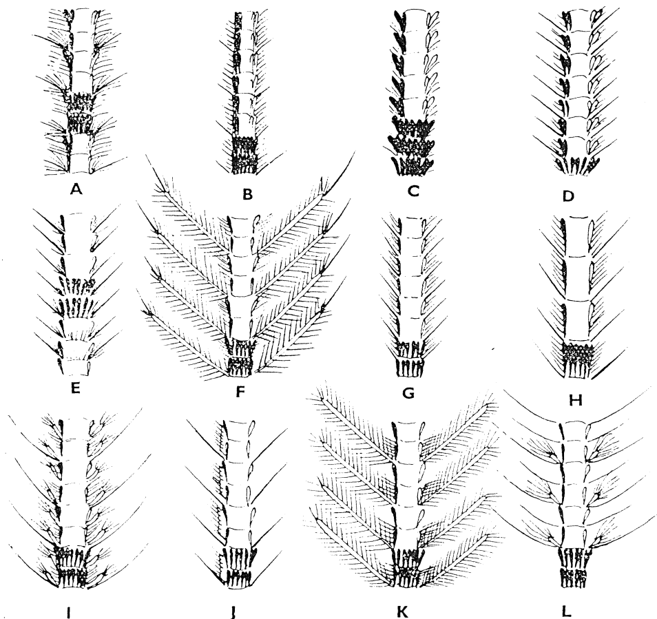
2. ábra. A: Hypena proboscidalis L., B: Bomolocha crassalis F., C: Schrankia humidalis DBLD., D: Sch. Kalchbergi STGR. ssp. orientalis STGR., E: Hypenodes taenialis HBN., F: Chytolitha cribrumalis HBN., G: Simplicia rectalis Ev., H: Zanclognatha grisealis SCHIFF., I: Z. tarsicristalis HS., J: Z. lunalis Sc. (oldalról), K: Macrochilo tentacularia L. és L: Herminia barbalis CL. hím csápostorok néhány ízének sematikus rajza (a könnyebb szemléltethetőség érdekében az ízeket fedő pikkelyeket csak néhány ízben ábrázoltuk). (Eredeti)
