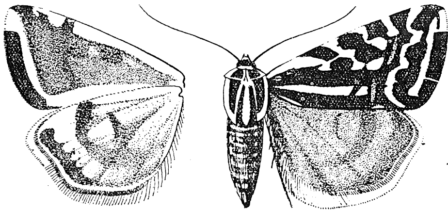
95. ábra. Emmelia trabealis Sc. ♀ (Eredeti)
