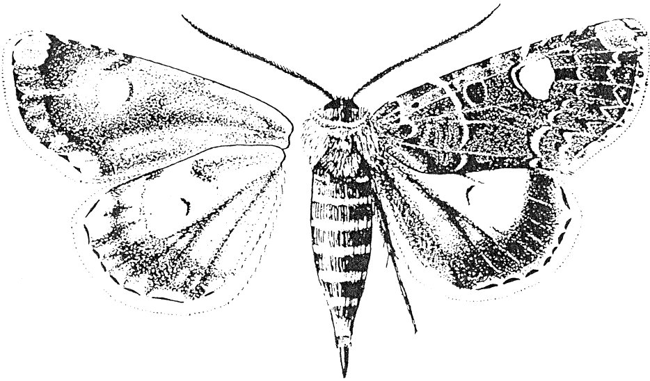
75. ábra. Oxytrypia orbiculosa Esp. ♀ (Eredeti).
