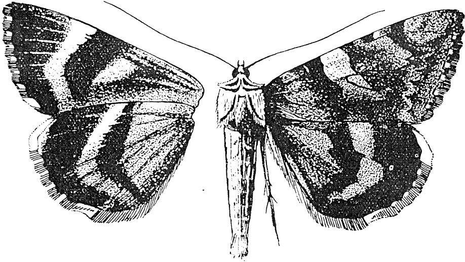
46. ábra. Catocala conversa ESP. ssp. agamos HBN. ♂ (Eredeti)
