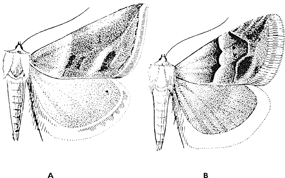
106. ábra. A: Porphyrinia noctualis HBN. ♂ és B: P. parva HBN. ♂ (Eredeti)
