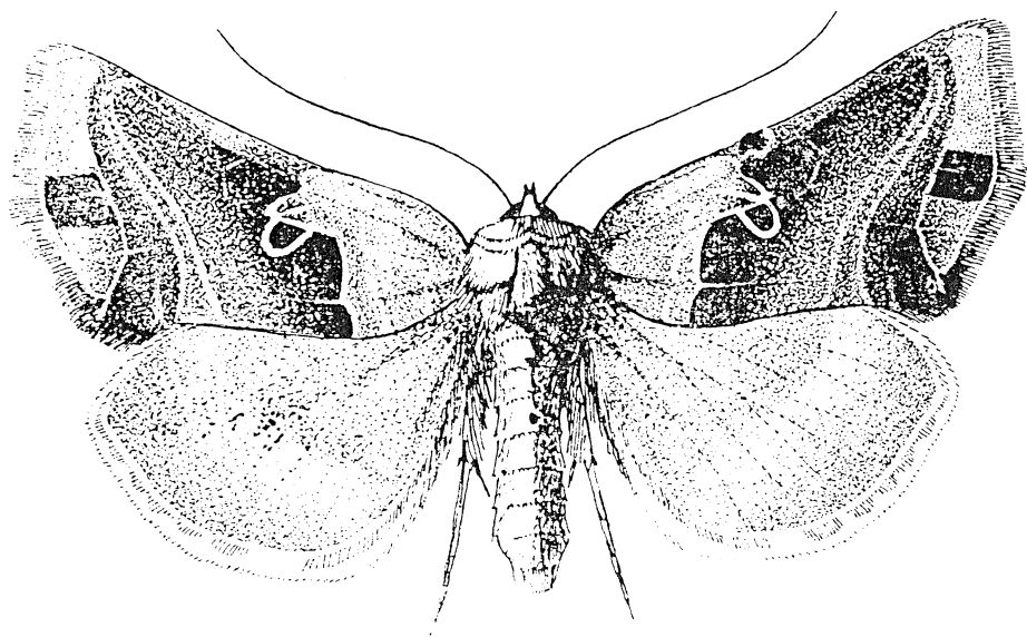
66. ábra. Eualcalia consona F. 5 (Eredeti)
